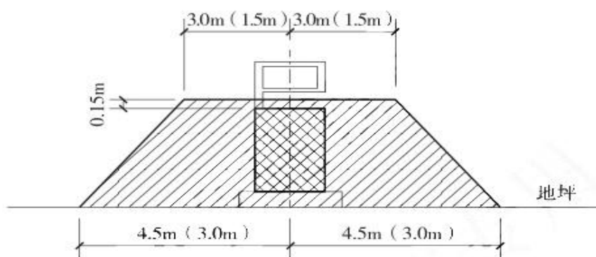
图 C.0.5 汽油加油机的爆炸危险区域划分
