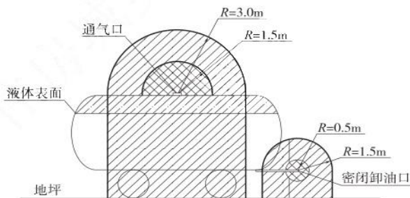
图 C.0.4 汽油油罐车的爆炸危险区域划分
