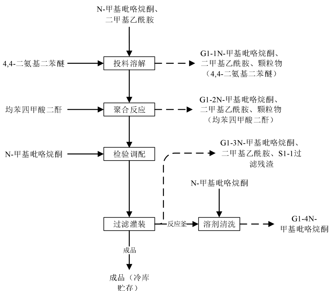
图 2.6.1-1 电机绝缘类聚酰亚胺树脂生产工艺流程图
