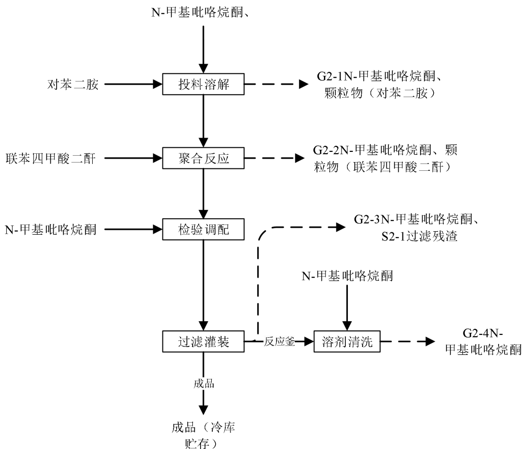
图 2.6.1-2 OLED 基材聚酰亚胺树脂生产工艺流程图
